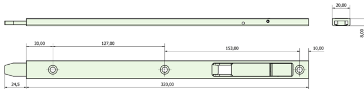
B84FLIP320
