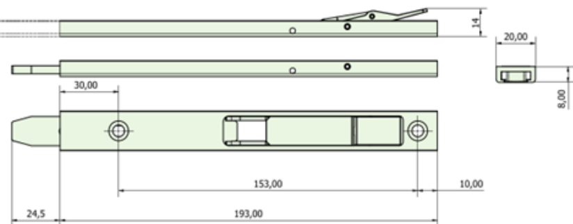
B84FLIP195
